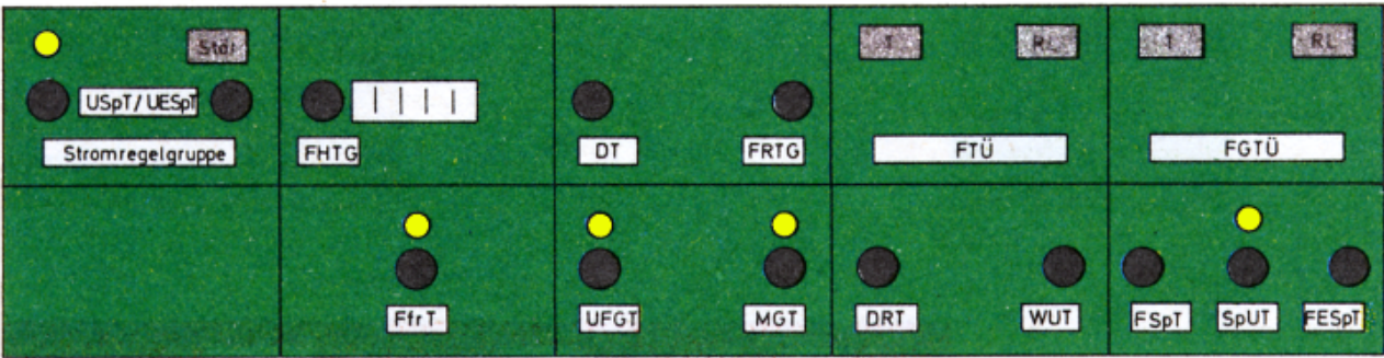
Fahrstraßen
